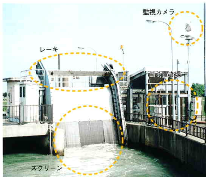
発電取水口（能美郡辰口町字宮竹地内）
