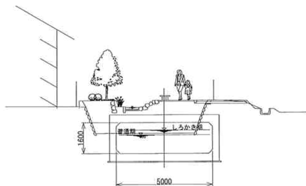
計 画 図
