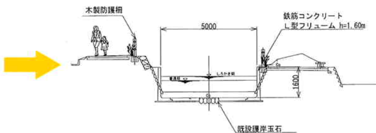
計 画 図
